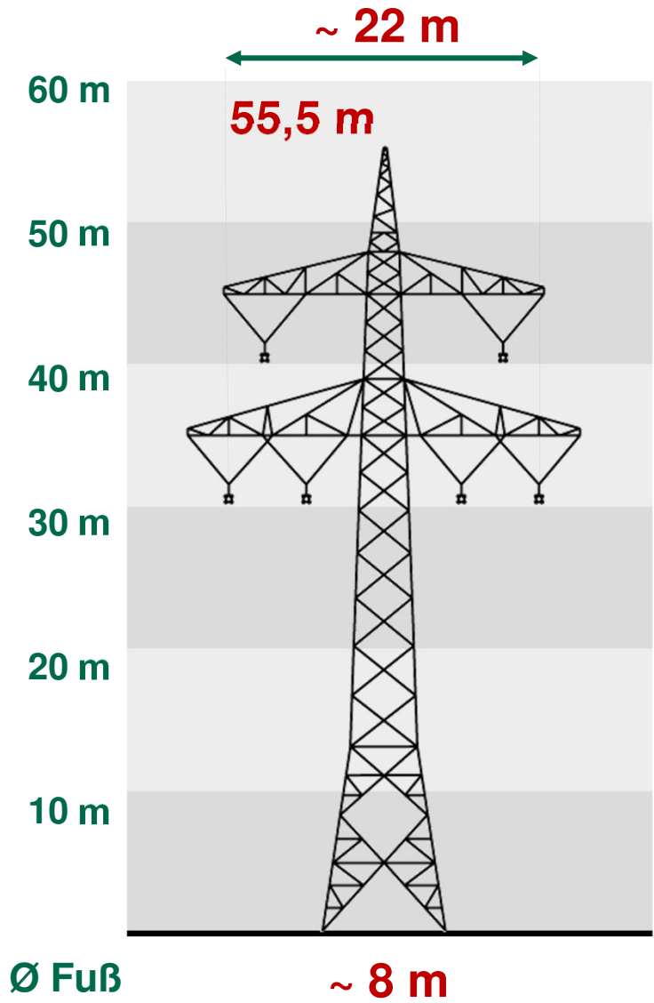
TenneT Vorschlag Gittermast
