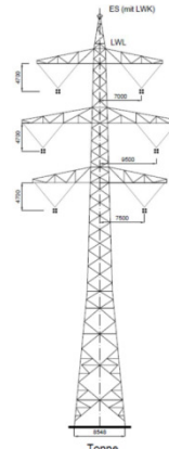
T3-Stahlgittermast 19m Trassenbreite
